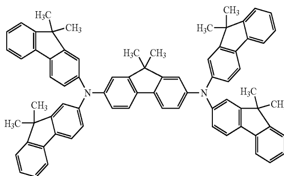
TFLEL
