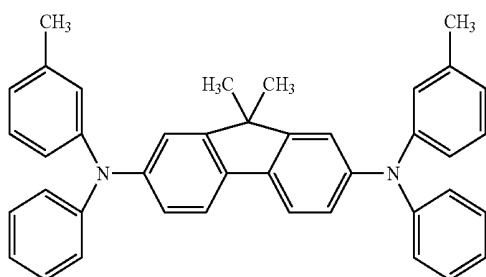
DTPDFL
