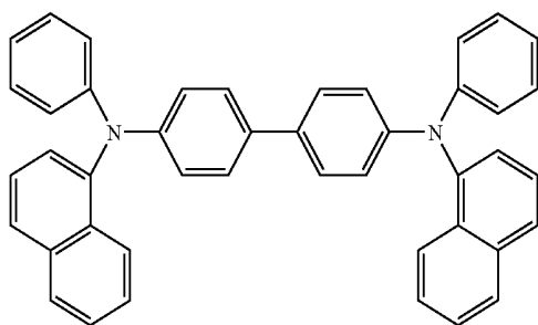
\alpha -NPD
