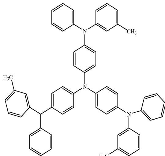
m-MTDATA
