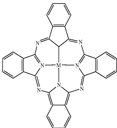
Pc-M
