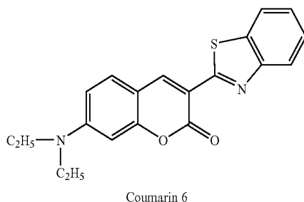
Coumarin 6
